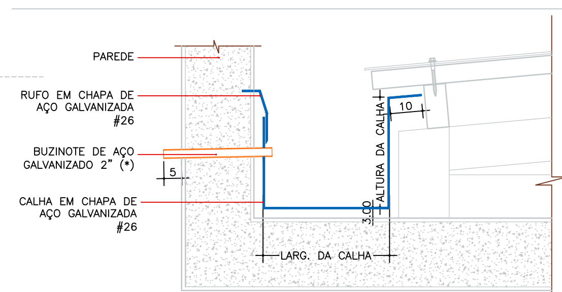
4 DETALHE - CALHA METÁLICA ESCALA 1:10
