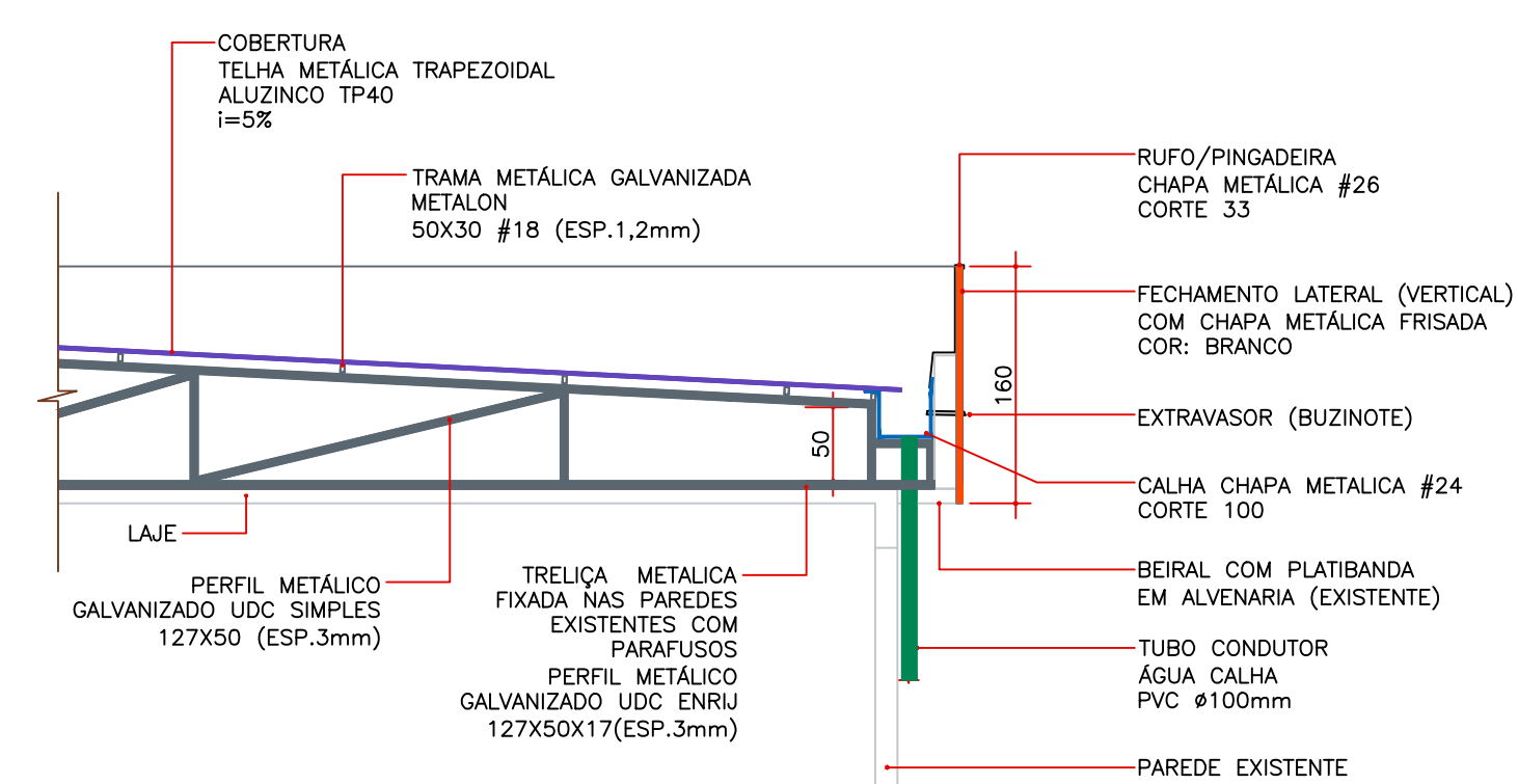
3 CORTE ESQUEMATICO
